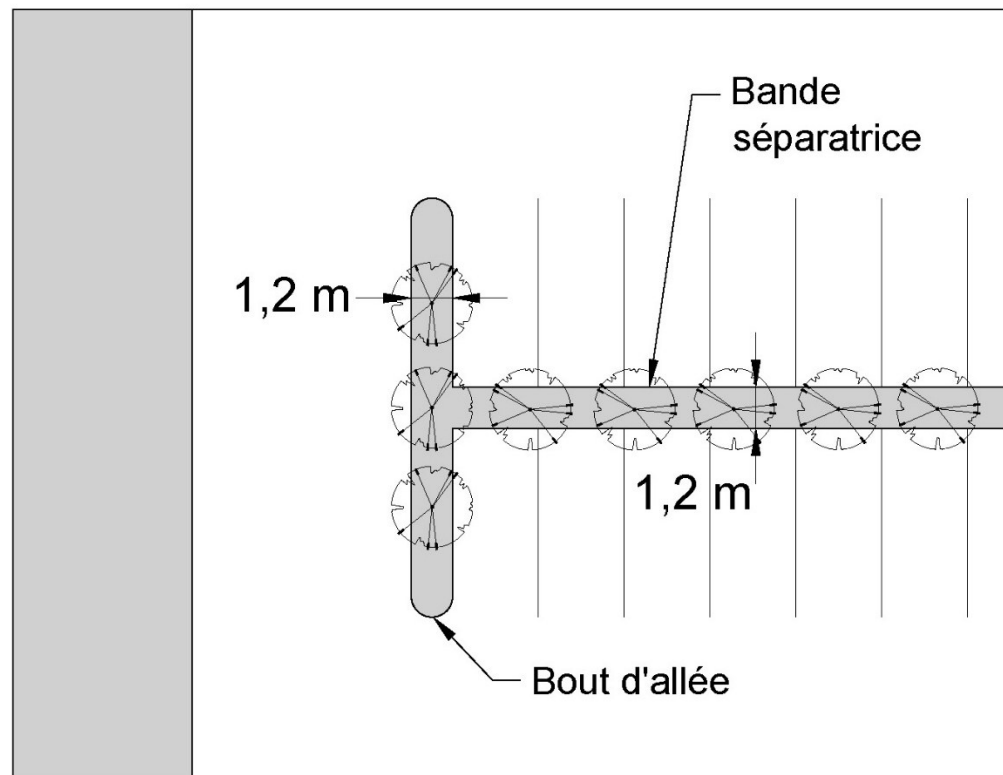
Figure 236. Aménagement d'un espace de stationnement comprenant 75 cases et plus
