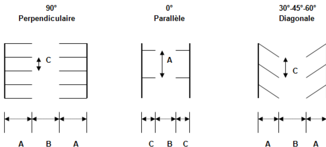
Figure 247. Dimensions d'une case de stationnement et d'une allée de circulation
