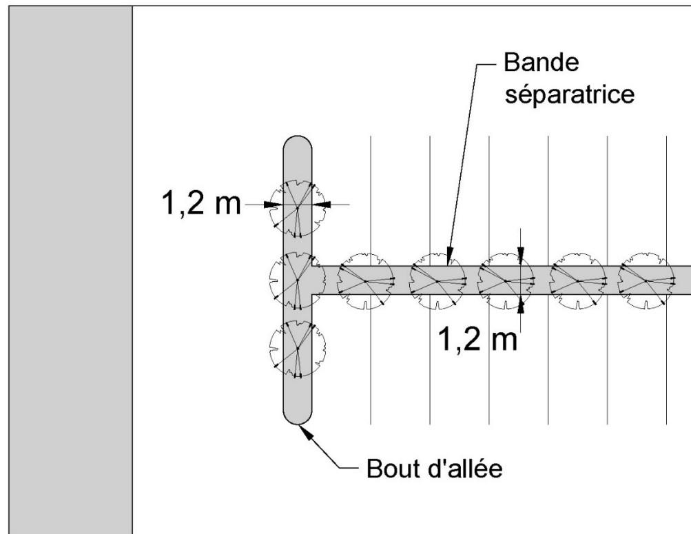
Figure 235. Aménagement d'un espace de stationnement comprenant 20 cases et plus
