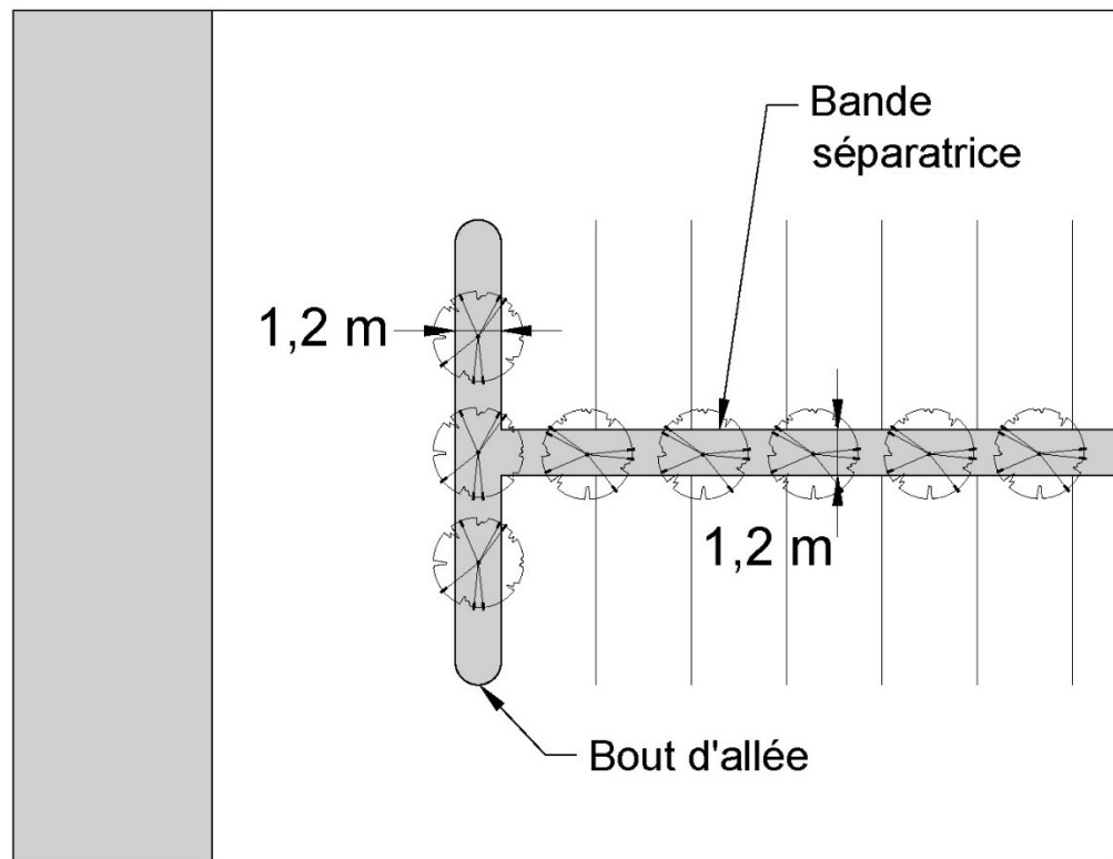
Figure 169. Aménagement d'un espace de stationnement extérieur pour une habitation comprenant 12 logements et plus
