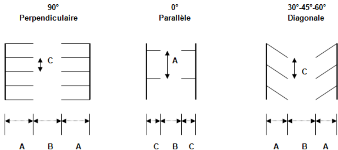
Figure 178. Dimensions d'une case de stationnement et d'une allée de circulation
